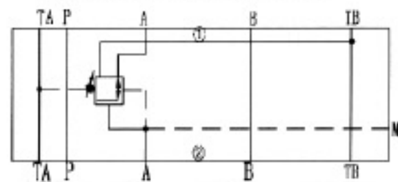
ZDR10DA...-50B/...YM...
