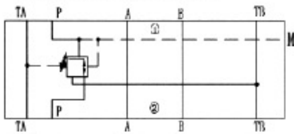
ZDR10DP...-50B/...YM...
