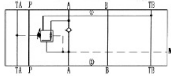
ZDR10DA...-50B/...Y...
